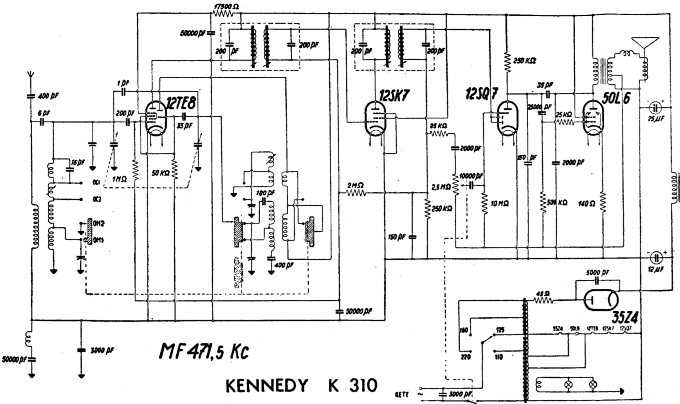
MAGNADYNE RADIO - Mod. KENNEDY K 310 - Onde medie divise e due gamme di onde corte. Media frequenza 471 kc. Potenza d'uscita 1,5 watt indistorti.
